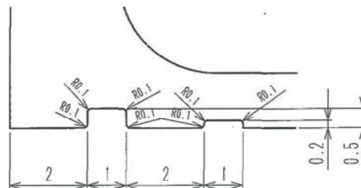
A部詳細 10/1
