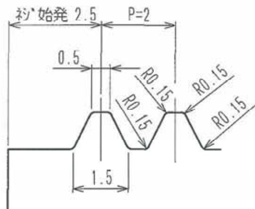
ネジ部詳細 10/1
